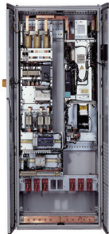
Пример внутренней компоновки SINAMICS G 150 исполнения "А"
